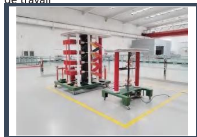
雷电冲击测试台 Lightning impulse test bench Banc d'essai d'impact de foudre
