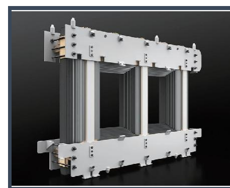
干变铁芯 Dry-type transformer iron core Noyau à changement sec
