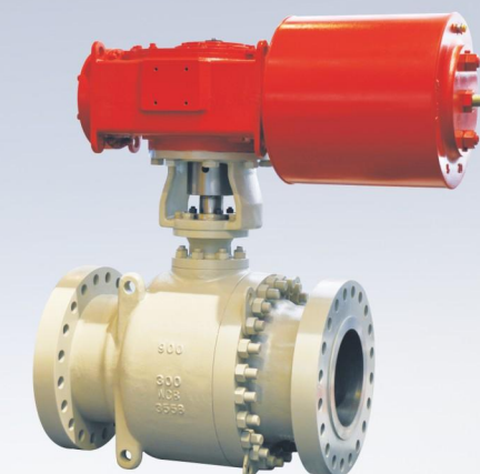
锁渣球阀 Slag Lock hopper Ball Valve
