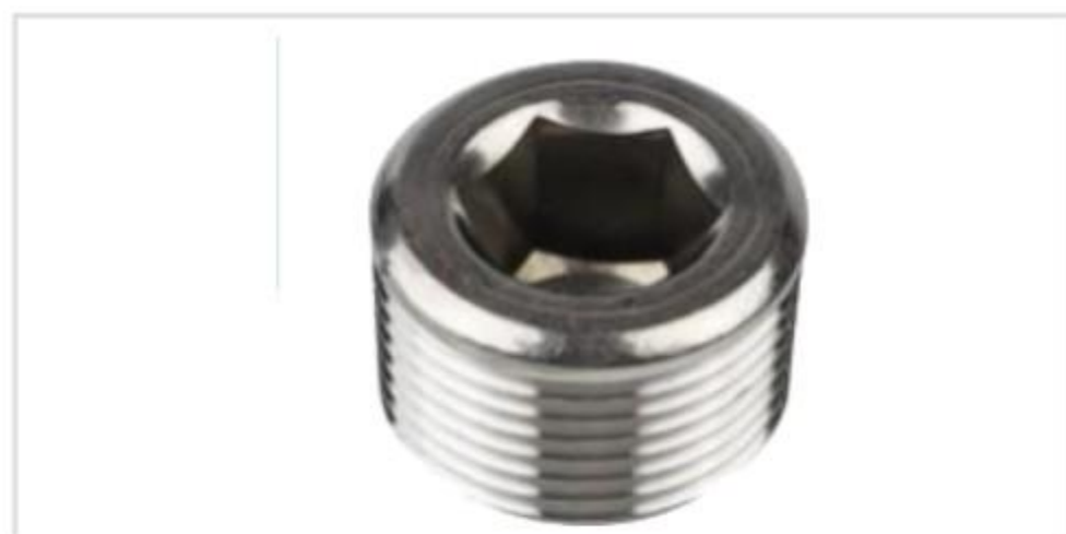
内六角塞头 Hexagonal plug head 材质:不锈钢201/304/316L/2205等 口径:1/8"-4"(DN6-DN100) 压力:PN1.6
