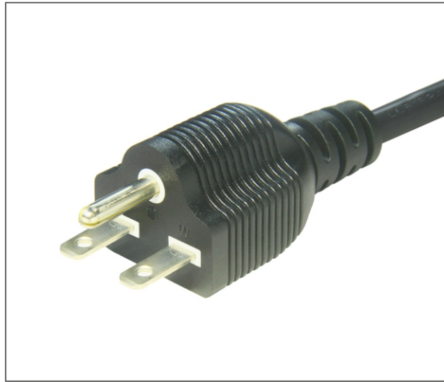
• NEMA 6-15P Plug
