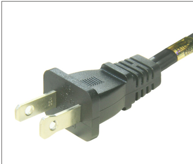
• NEMA 1-15P 2Pin Plug
