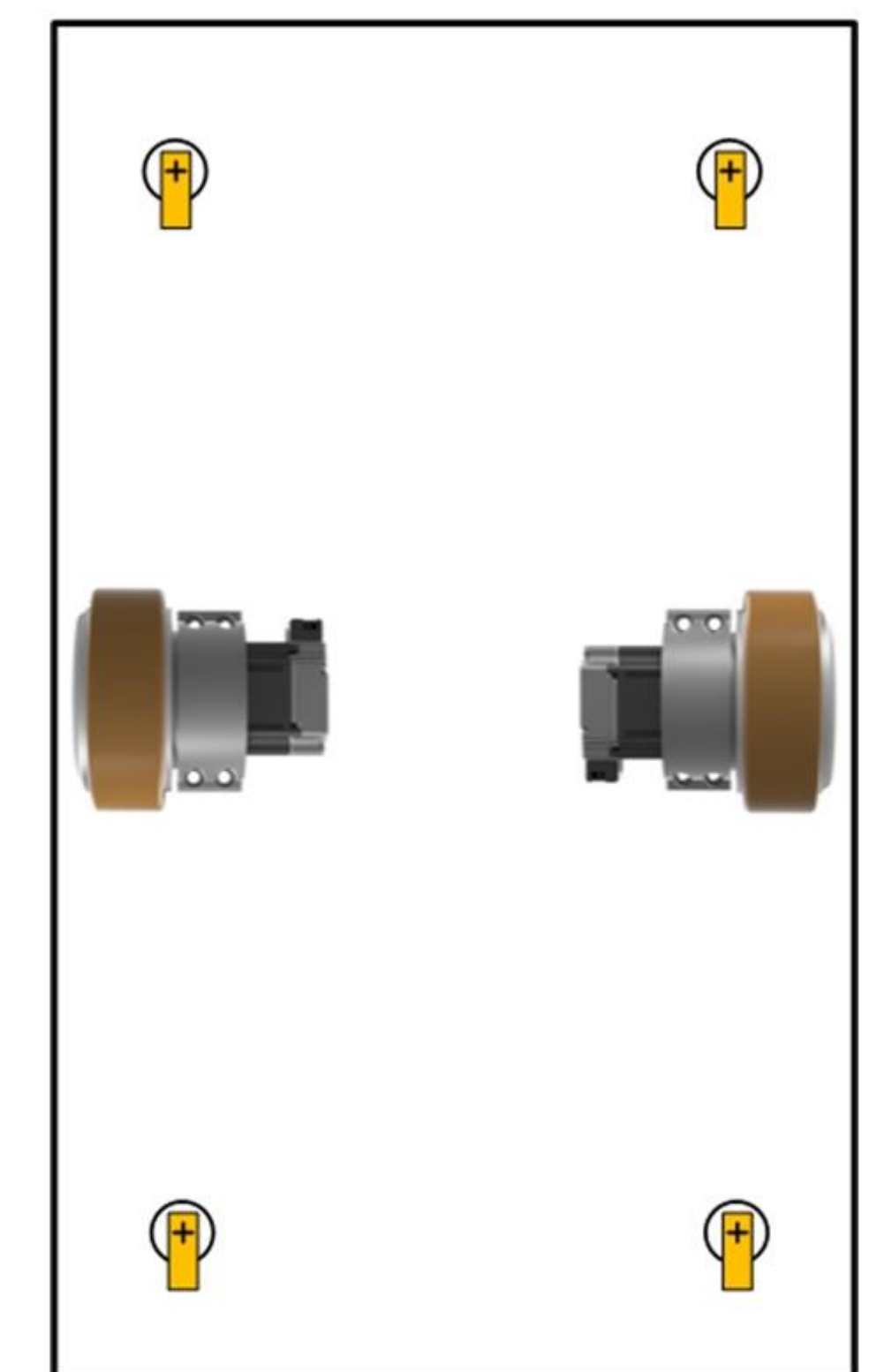
中轴差速轮
