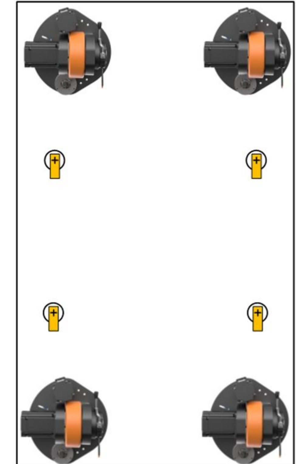
四舵轮
