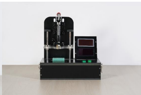
耳机 PCBA 测试治具 Headphone PCBA test fixture
