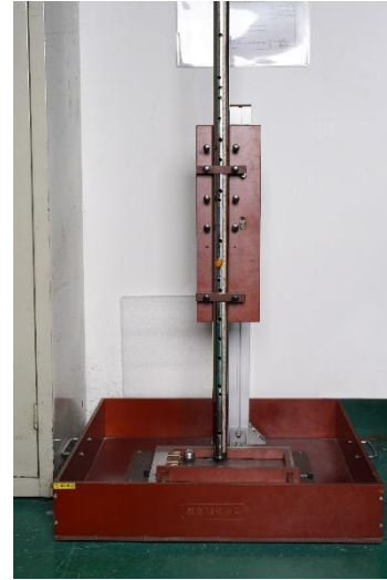
钢球冲击试验台 Steel ball impact test bench
