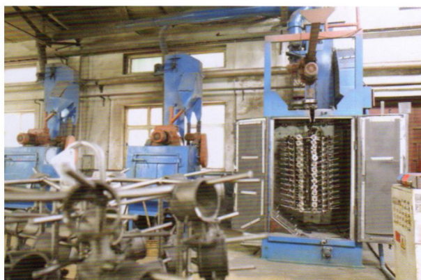
抛丸 Blasting
