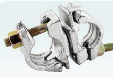
RFH-A015 德式防滑旋转扣件 German Type Swivel Coupler 48.3mm 1.40kg
