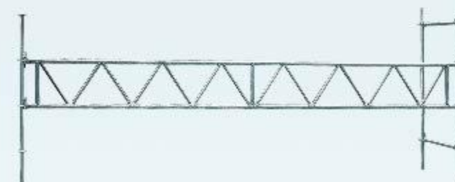
RFH-B001K1 三角架(mm) Bracket 732/5.85kg
