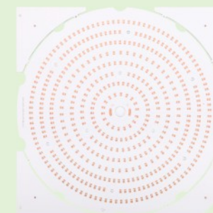
高压铝基板 High Voltage MCPCB
