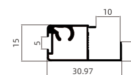
WZB-116 极简移门上方 Minimalist Sliding Door Upper Rail
