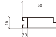
NBW-72 后扣板 Rear Snap Panel
