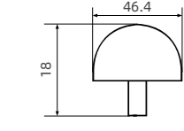
GT18-032 46 圆弧层板条 46 Arc Shelf Strip
