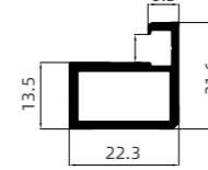
FY-A085 20 框小边 20 Frame Edges
