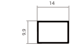
PC-14X10 方管 10x14 Square Tube.
