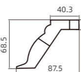
NBW-003 顶线 Top Line
