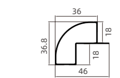
壁厚 Thickness:0.8mm 米重 Weight:0.304kg/m
