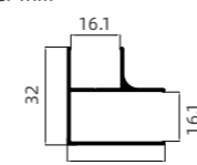
PC-G-098 16 转角料 16 Corner Trim
