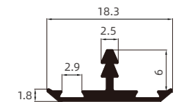
G-084 18 厘铝封边条 18mm Aluminum Edge Banding
