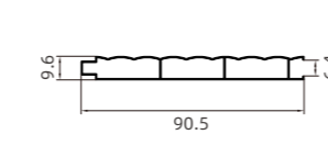
NBW-114 波浪板 Wave Panel.
