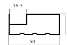
NBW-004 罗马柱 1 Roman Column 1
