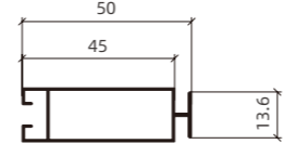
NBW-73 小扣板 Small Snap Panel
