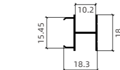
壁厚 Thickness:0.8mm 米重 weight:0.12kg/m
