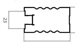
A-081 61 门框 61 Door Frame
