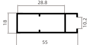
NBW-335 55 平板门框 55mm Flat Door Frame
