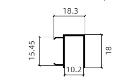
壁厚 Thickness:0.8mm 米重 weight:0.121kg/m
