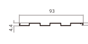
NBW-578 5 厘格栅板 5mm Grille Panel
