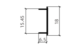
壁厚 Thickness:0.8mm 米重 weight:0.059kg/m
