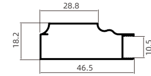
G-23 46 门扇 46mm Door Leaf.
