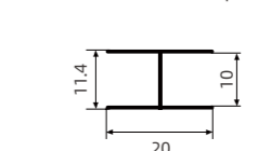
壁厚 Thickness:0.8mm 米重 weight:0.115kg/m
