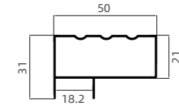
G-072 卡 18 厘罗马柱 Snap-on 18mm Roman column.
