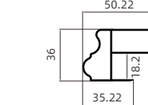
NBW-255 18 厘 255 小顶线 18mm 255 Small Crown Molding
