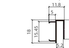
壁厚 Thickness:0.8mm 米重 weight:0.11kg/m
