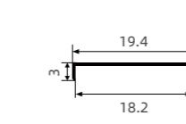
壁厚 Thickness:0.8mm 米重 weight:0.044kg/m
