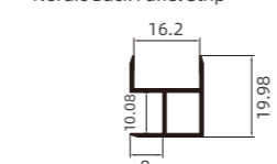
NBW-346 北欧背板条 Nordic Back Panel Strip
