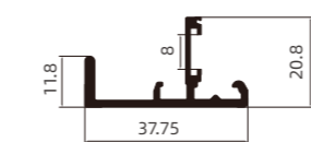
FY-A097 卡 5 厘免开铰链孔 F 款拉手 Snap-on 5mm Hinge Hole-Free F-Style Pull Handle.
