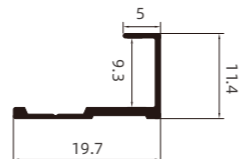
HQB-006 收口 Edge Finishing
