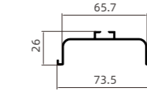
HW-1268 中柜拉手 Middle Cabinet Pull Handles
